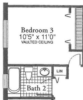
OPTIONAL BEDROOM 3
