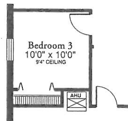
OPTIONAL BEDROOM 3
